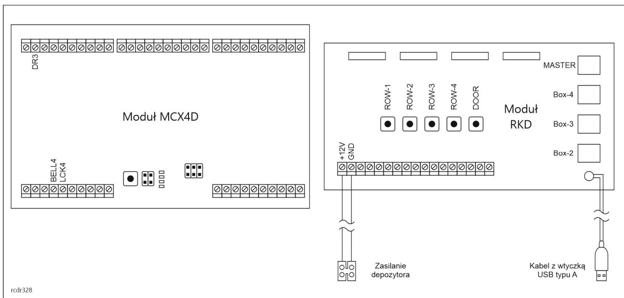
Rys. 8 Moduły RKD i MCX4D
