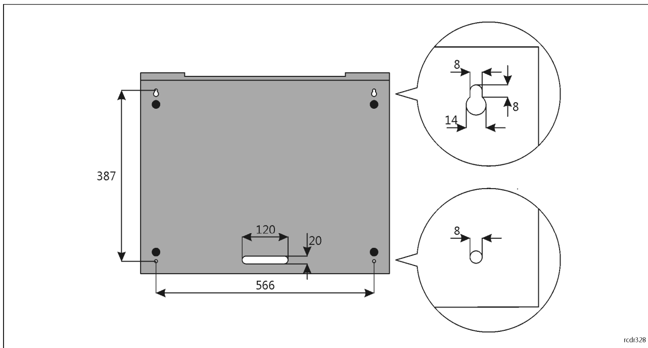
Rys. 5 Pokrywa tylna depozytora
