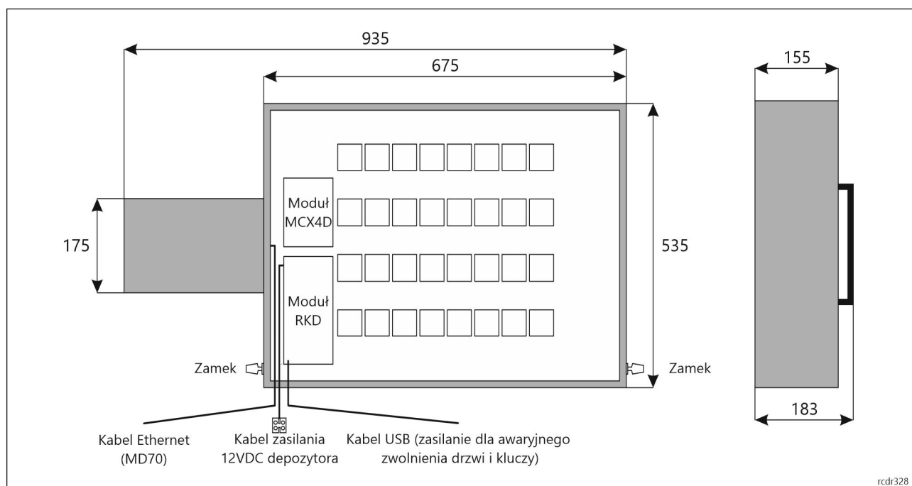
Rys. 4 Wnętrze depozytora po zdjęciu pokrywy tylnej
